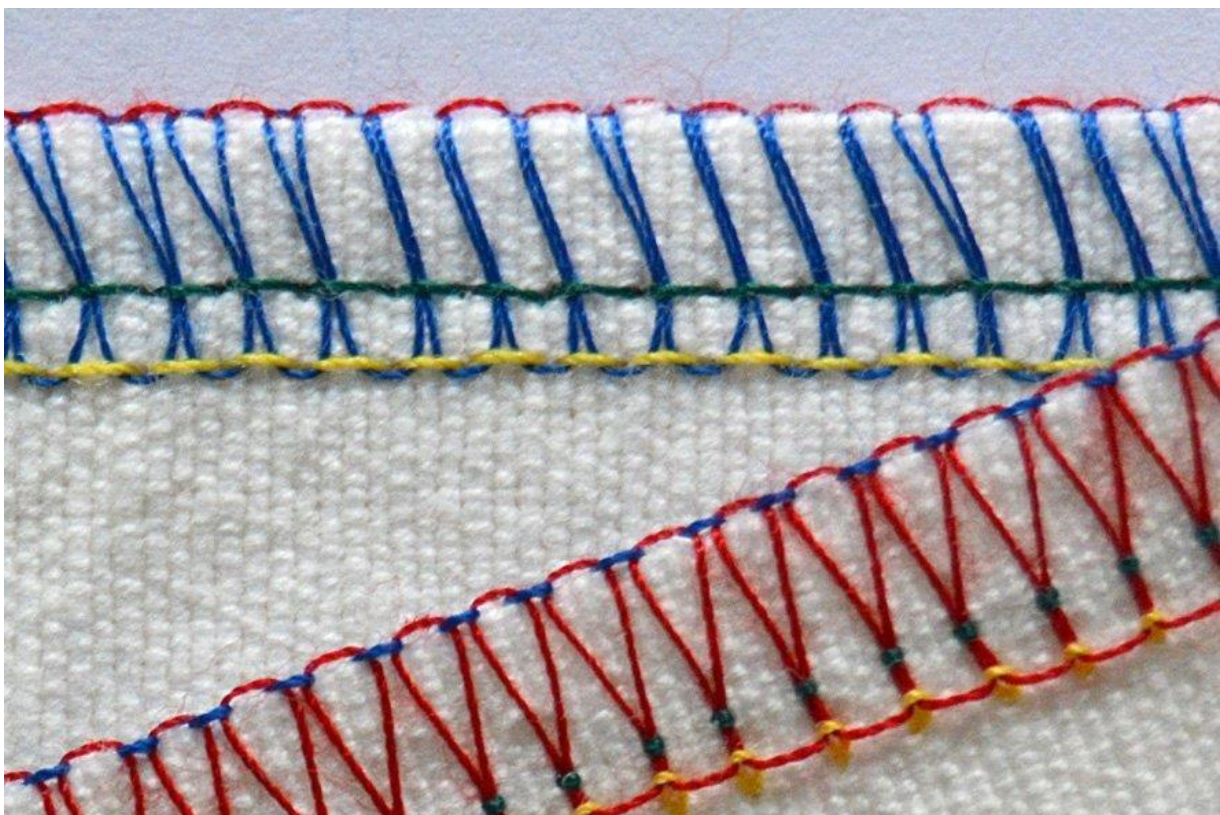
Beispiel für eine Overlock- bzw. Endelnaht (Quelle Bernina – Fach-Nähmaschinen)
