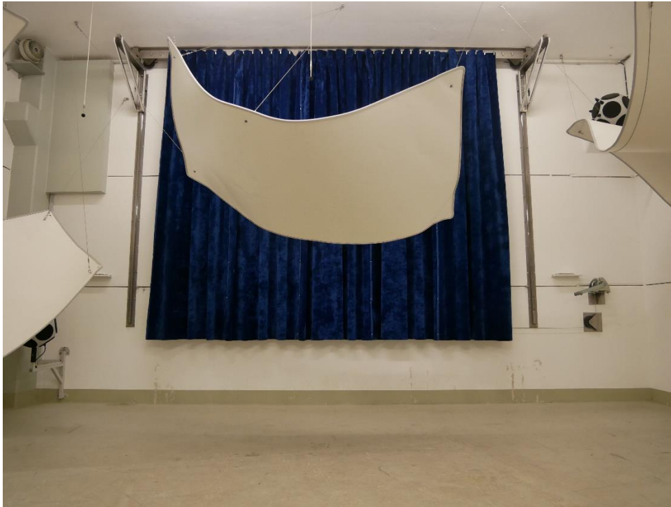
Abbildung B.1. Prüfanordnung im Hallraum (frontale Ansicht).
